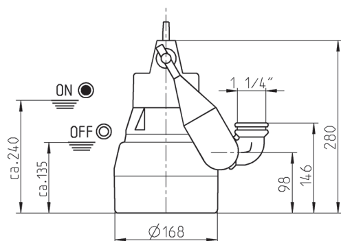
Hauptmaße und Schalthöhen U5KS (mm)
