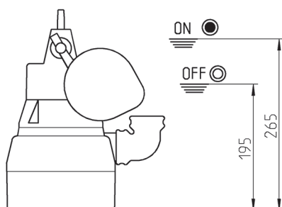
Hauptmaße und Schalthöhen Sonderschwimmer (mm)
