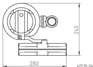
Hauptmaße und Schalthöhen GR 32 (mm)
