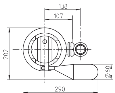
Hauptmaße und Schalthöhen Sonderschwimmer (mm)
