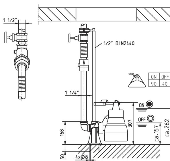
Hauptmaße und Schalthöhen GR 32 (mm)
